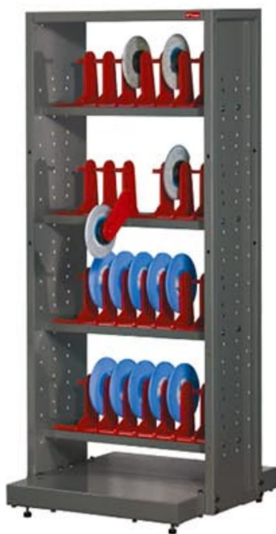
GR-6558 (118-03) 653W x 600D x 1460H mm
